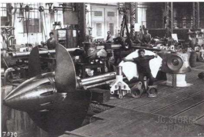
Pohled do výroby Kaplanových turbín ve firmě Ignác Starek.
